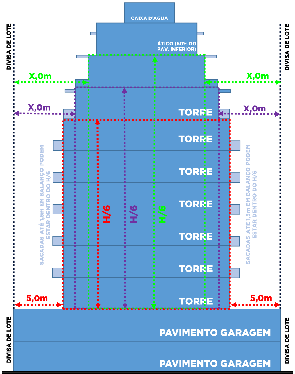
TORRE COM ESCALONAMENTO
